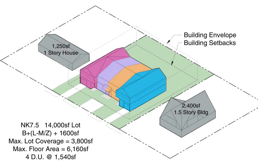
NK7.5 B+(L-M/Z) + 1600sf M.H. Allowance
